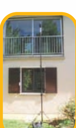
Microphone (ici placé à une hauteur d'environ 4 m) : enregistre les fluctuations des niveaux de bruit
